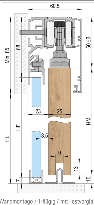
Wandmontage / 1-flügelig
