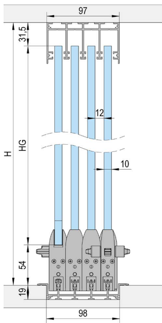
Beépítés süllyesztett felső sínrel / 4 szárnyú sínrel
