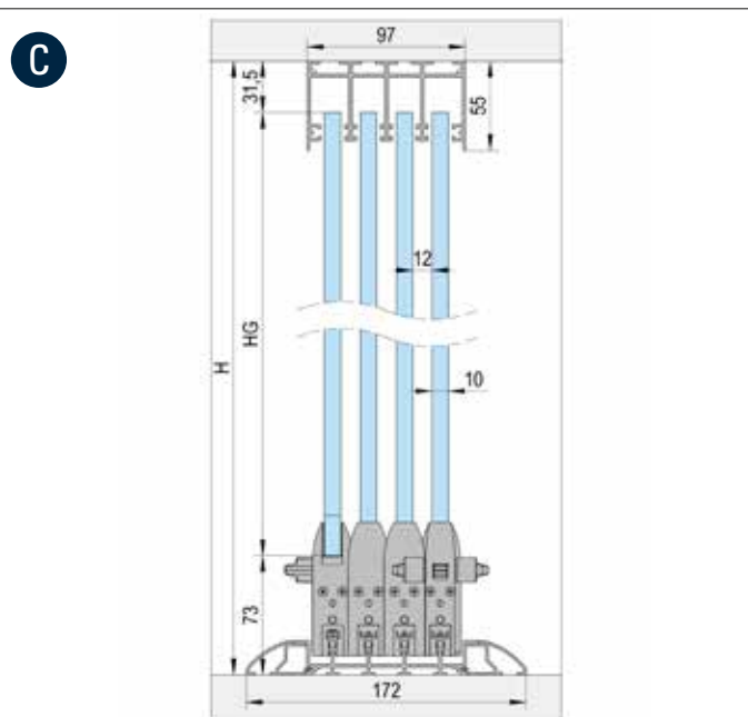
Montage mit eingelassener Laufschiene mit Rampe / 4-flügelig
