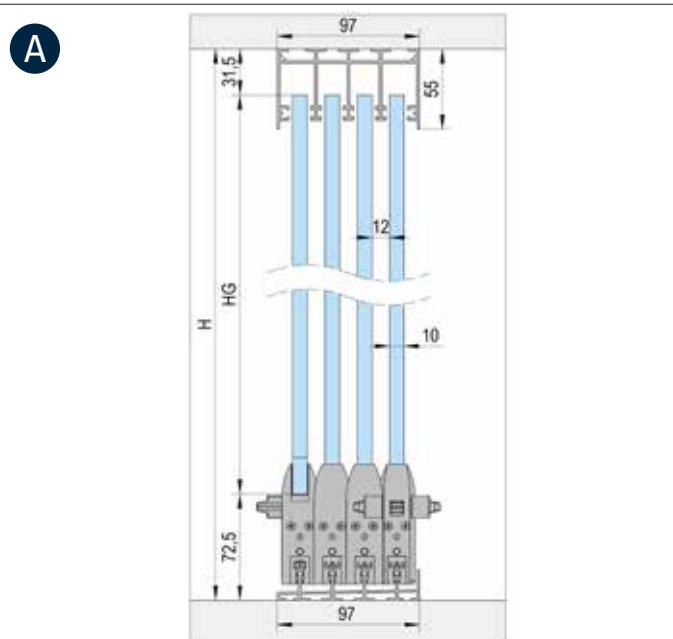
Montage mit aufgesetzter Laufschiene / 4-flügelig
