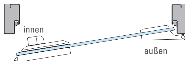
Bedienknebel auf Klemmplatenseite (DIN rechts auswärts)
