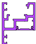
Zargenprofil
